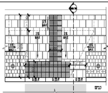
תכנית קנ"מ 1:50 מזדקל רחבה 0-3.0 מ
