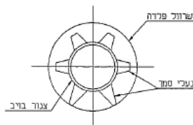
חתך א-א
