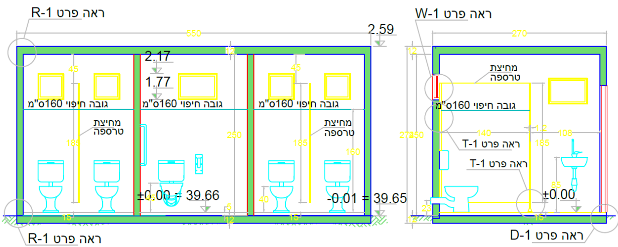
חתך 2-2
